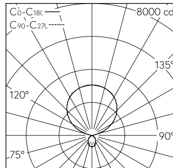
LED 2700 – 6500 K 83 W 9870 lm-h / CIE Flux 66 92 98 12 100 / D63 nach DIN 5040
