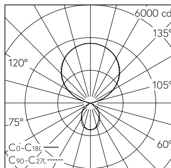
LED 2700 – 6500 K 96 W 12980 lm-h / CIE Flux 66 92 98 21 100 / D63 nach DIN 5040
