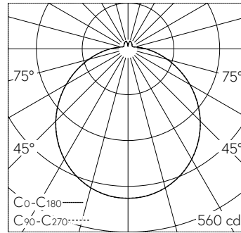
LED 2700 K 19.6 W 1588 lm-h / CIE Flux 43 73 90 91 100 / A31 nach DIN 5040
