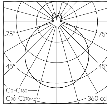
LED 3000 K 10 W 1040 lm-h / CIE Flux 45 75 92 86 100 / B42 nach DIN 5040
