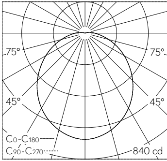
LED 3000 K 28.5 W 2131 lm-h / CIE Flux 45 75 91 96 100 / A40 nach DIN 5040
