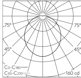
LED 3000 K 3,0 W 319 lm-h / CIE Flux 45 75 91 96 100 / A40 nach DIN 5040
