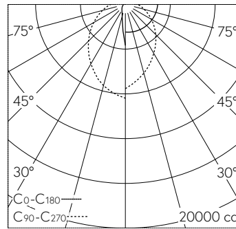
LED 3000 K 51 W 4542 lm-h / A81 nach DIN 5040
