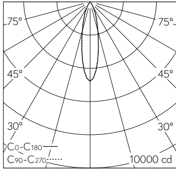
LED 23.5 W 1301 lm-h 24° / CIE Flux 99 100 100 100 100 / A80 nach DIN 5040
