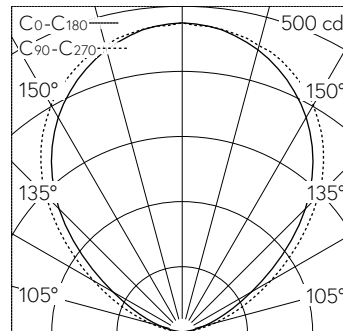
LED 3000 K 12.5 W 1120 lm-h / CIE Flux 0 0 0 100 / E83 nach DIN 5040
