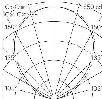
LED 4000 K 19,1 W 1907 lm-h / CIE Flux 0 0 0 100 / E83 nach DIN 5040
