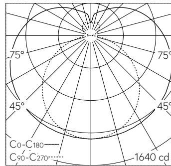
LED 3000 K 73 W 8108 lm-h / CIE Flux 34 61 82 69 100 / B21 nach DIN 5040
