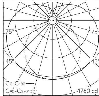
LED 4000 K 73 W 8575 lm-h / CIE Flux 34 61 82 69 100 / B21 nach DIN 5040
