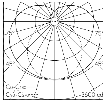
LED 4000 K 147 W 16739 lm-h / CIE Flux 34 61 82 69 100 / B21 nach DIN 5040
