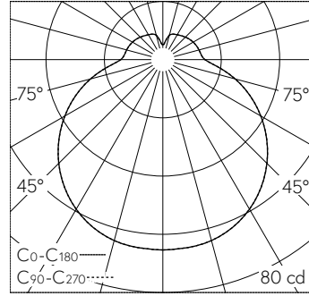
LED 3000 K 3,0 W 319 lm-h / CIE Flux 38 67 87 77 100 / B32 nach DIN 5040
