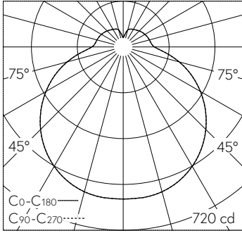
LED 3000 K 33.5 W 2822 lm-h / CIE Flux 39 68 88 79 100 / B32 nach DIN 5040
