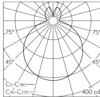
LED 4000 K 13.3 W 1310 lm-h / CIE Flux 43 73 91 77 100 / B32 nach DIN 5040
