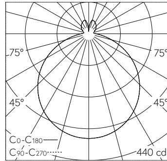
LED 4000 K 13.3 W 1290 lm-h / CIE Flux 45 76 93 86 100 / B43 nach DIN 5040
