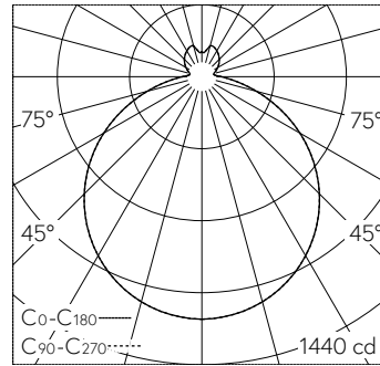
LED 4000 K 35 W 4330 lm-h / CIE Flux 45 75 92 85 100 / B43 nach DIN 5040
