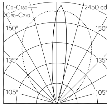
LED RGBW 0 K 28 W 1235 lm-h / CIE Flux 0 0 2 0 100 / E84 nach DIN 5040
