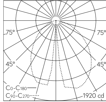
LED 4000 K 31.5 W 2294 lm-h 15° / CIE Flux 54 84 97 98 100 / A51 nach DIN 5040
