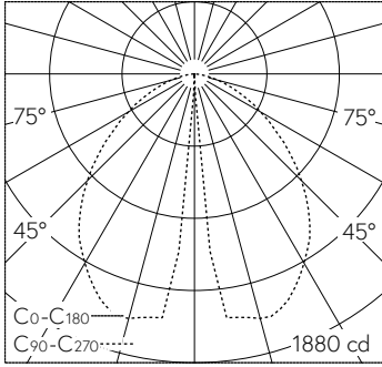
LED 4000 K 31.5 W 2368 lm-h 0° / CIE Flux 55 85 97 98 100 / A51 nach DIN 5040
