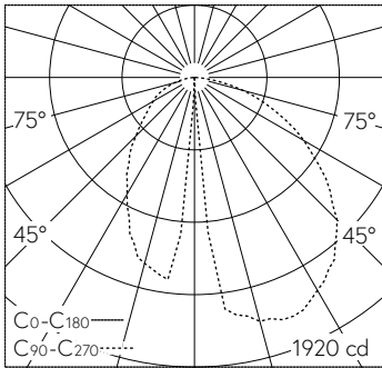
LED 4000 K 31.5 W 2203 lm-h 30° / CIE Flux 51 81 96 98 100 / A41 nach DIN 5040
