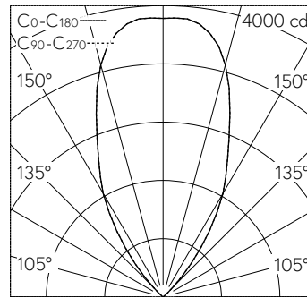
LED 4000 K 30 W 3113 lm-h 54° / E84 nach DIN 5040
