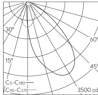
LED O K 45 W 2239 lm-h / CIE Flux 69 95 99 100 100 / A60 nach DIN 5040
