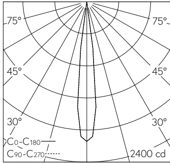
LED O K 18 W 196 lm-h 13.0°_Spot / CIE Flux 100 100 100 100 100 / A80 nach DIN 5...
