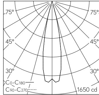
LED 18 W 196 lm-h 22°_Flood / CIE Flux 100 100 100 100 100 / A80 nach DIN 5040
