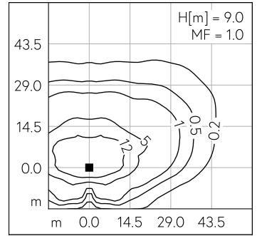
LED 4000 K 103 W 14866 lm-h H = 9 m / CIE Flux 32 65 92 100 100 / A20 nach DIN ...
