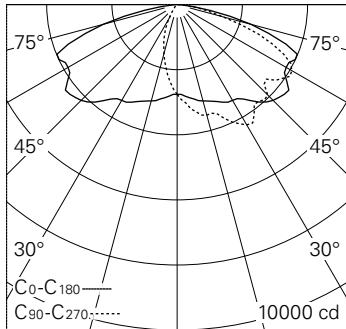
LED 4000 K 103 W 14866 lm-h H = 10 m / CIE Flux 32 65 92 100 100 / A20 nach DI...
